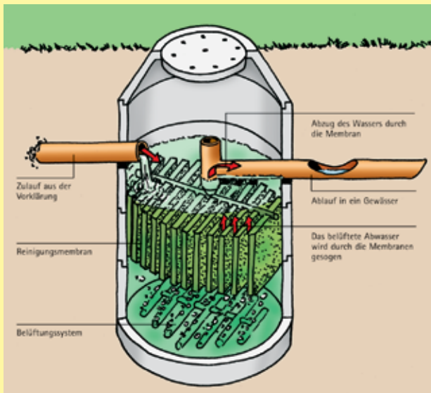
Abbildung 8: Belebungsanlage mit Membranfiltration [13]
