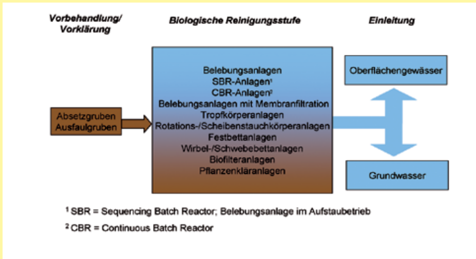
Abbildung 1: Übersicht über Kleinkläranlagen-Verfahrensvarianten
