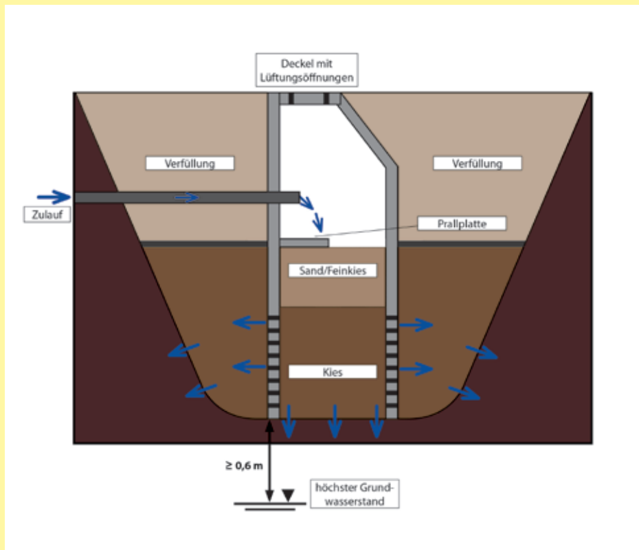
Abbildung 15: Prinzipskizze einer Versickerungsgrube mit Schacht, verändert nach [6]
