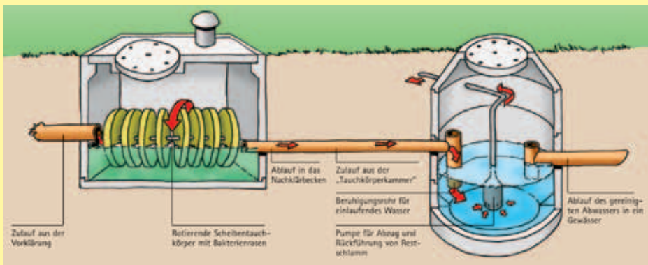
Abbildung 10: Rotations-/Scheibentauchkörperanlage [13]
