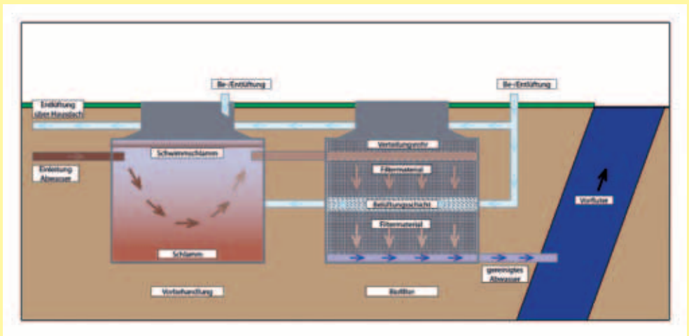
Abbildung 5: Biofilteranlage
