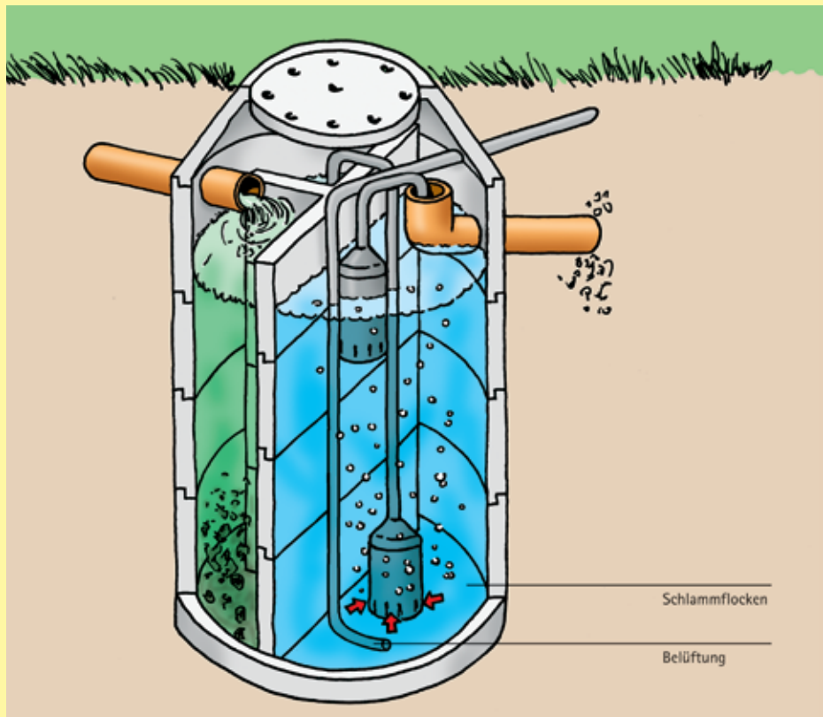
Abbildung 13: Nachrüstsatz einer SBR-Anlage [13]
