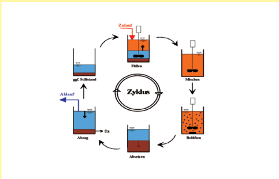
Abbildung 7: Zyklus einer SBR-Anlage
