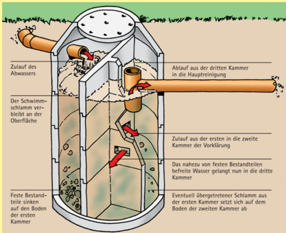
Abbildung 2: Mehrkammerausfallgrube mit Durchtrittsöffnungen [13]
