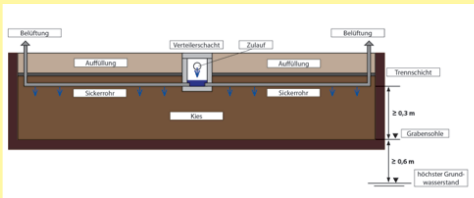
Abbildung 14: Prinzipskizze eines Versickerungsgrabens, verändert nach [6]
