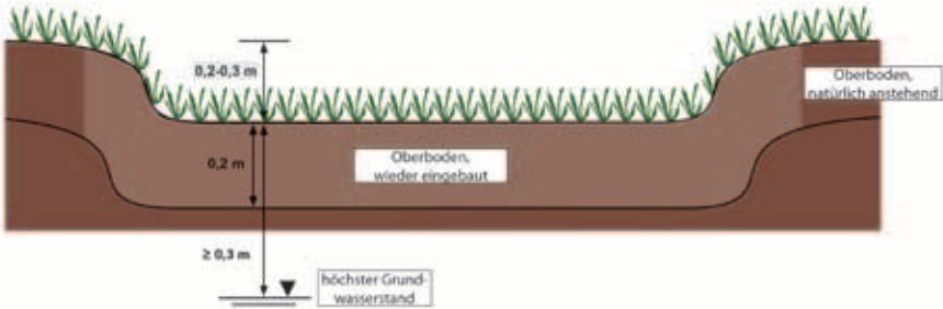
Abbildung 16: Prinzipskizze einer Versickerungsmulde, verändert nach [6]
