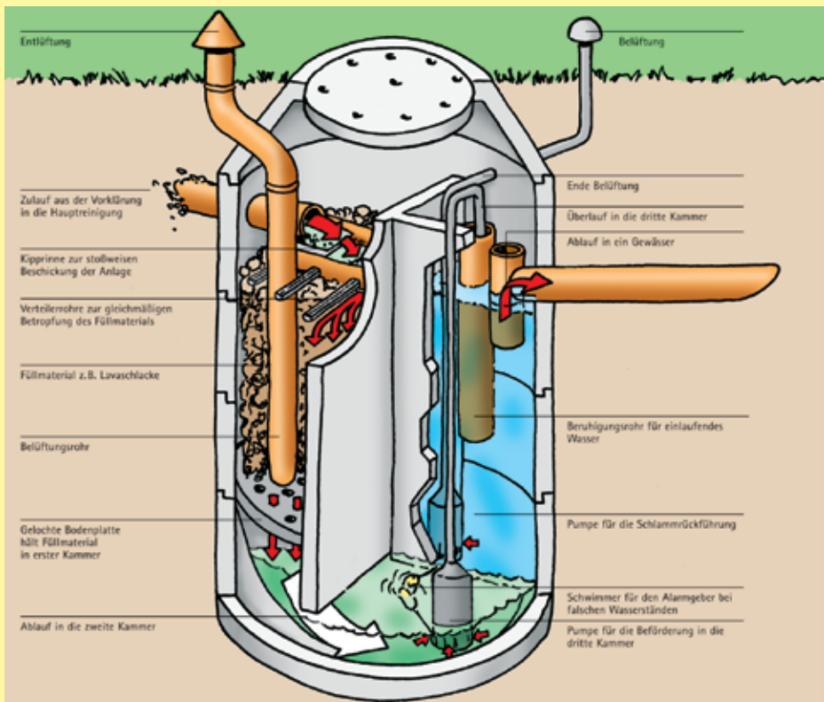
Abbildung 9: Tropfkörperanlage [13]
