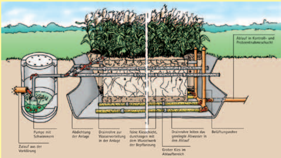
Abbildung 4: Vertikal durchflossene Pflanzenkläranlage [13]
