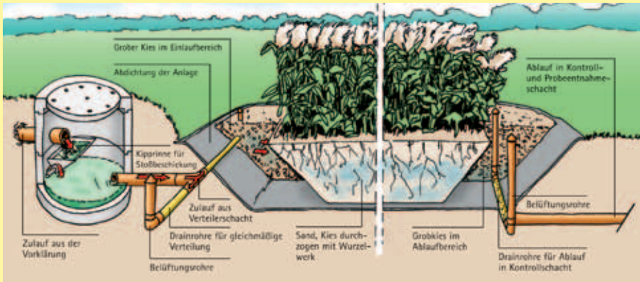
Abbildung 3: Horizontal durchflossene Pflanzenkläranlage [13]
