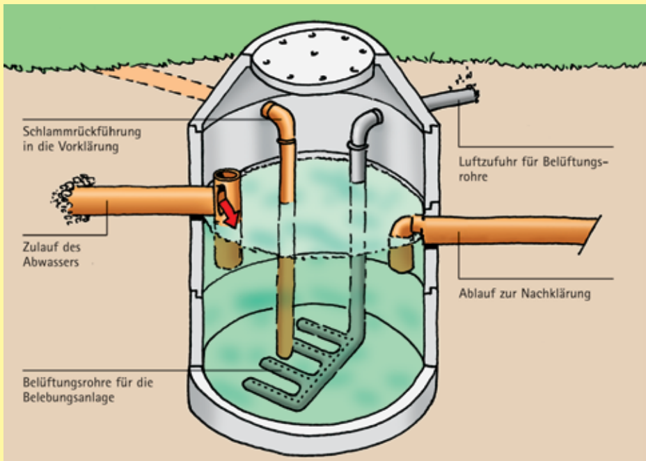
Abbildung 6: Belebungsbecken [13]
